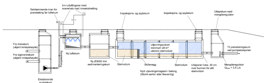
Figur 1: En skjematisk illustrasjon som viser prosessarrangementet. Tilbudstegning GH042 er hentet fra konkurransegrunnlag datert 15.03.2018.
