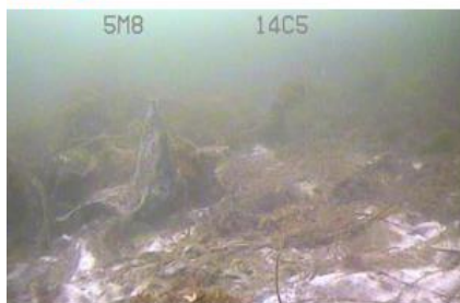
Figur 18. Typisk bilde av sjøbunnen mellom 3-6 m dybde. Sjøbunnen her er en blanding av bløtbunn og hardbunn. På bildet har makroalger slått seg til på steiner, mens områdene rundt er bløtbunn. Bildet viser at mye død plantemateriale sedimenteres og akkumuleres på sjøbunnen.
