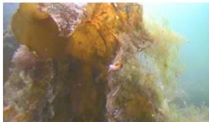
Figur 17. Typisk tareblad fra Bildøystraumen. Tarebladene var preget av begroing av trådformede alger.
