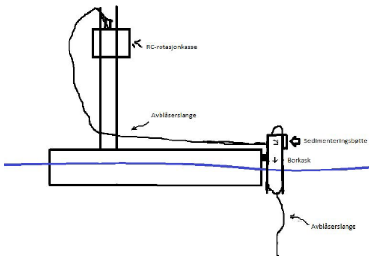
Figur 1: Boreslam går fra RC- rotasjonskassen og blir ledet ned til sjøbunnen gjennom avblåserlangen via sedimenteringsbøtten
