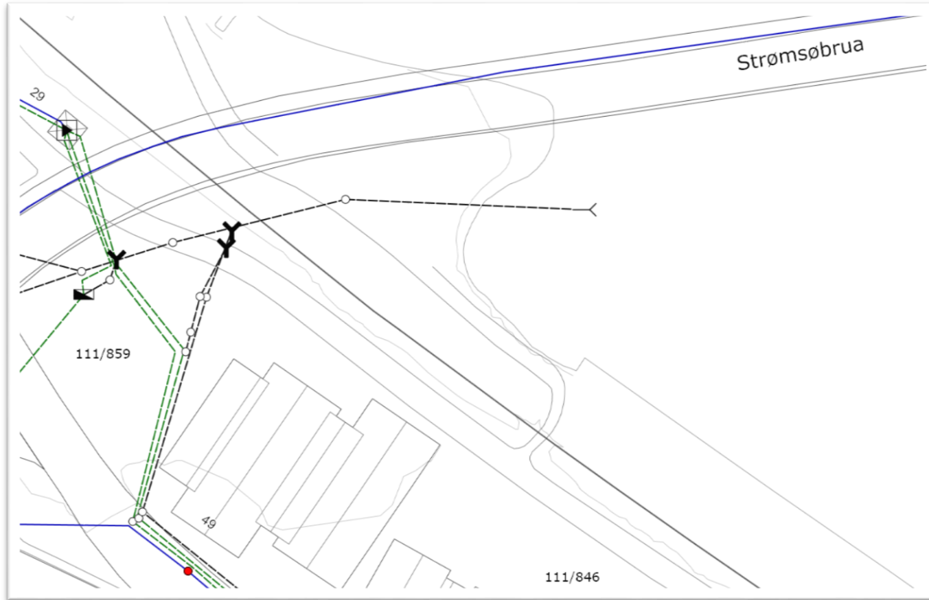
Figur 5 Overvannsledning med utslipp
