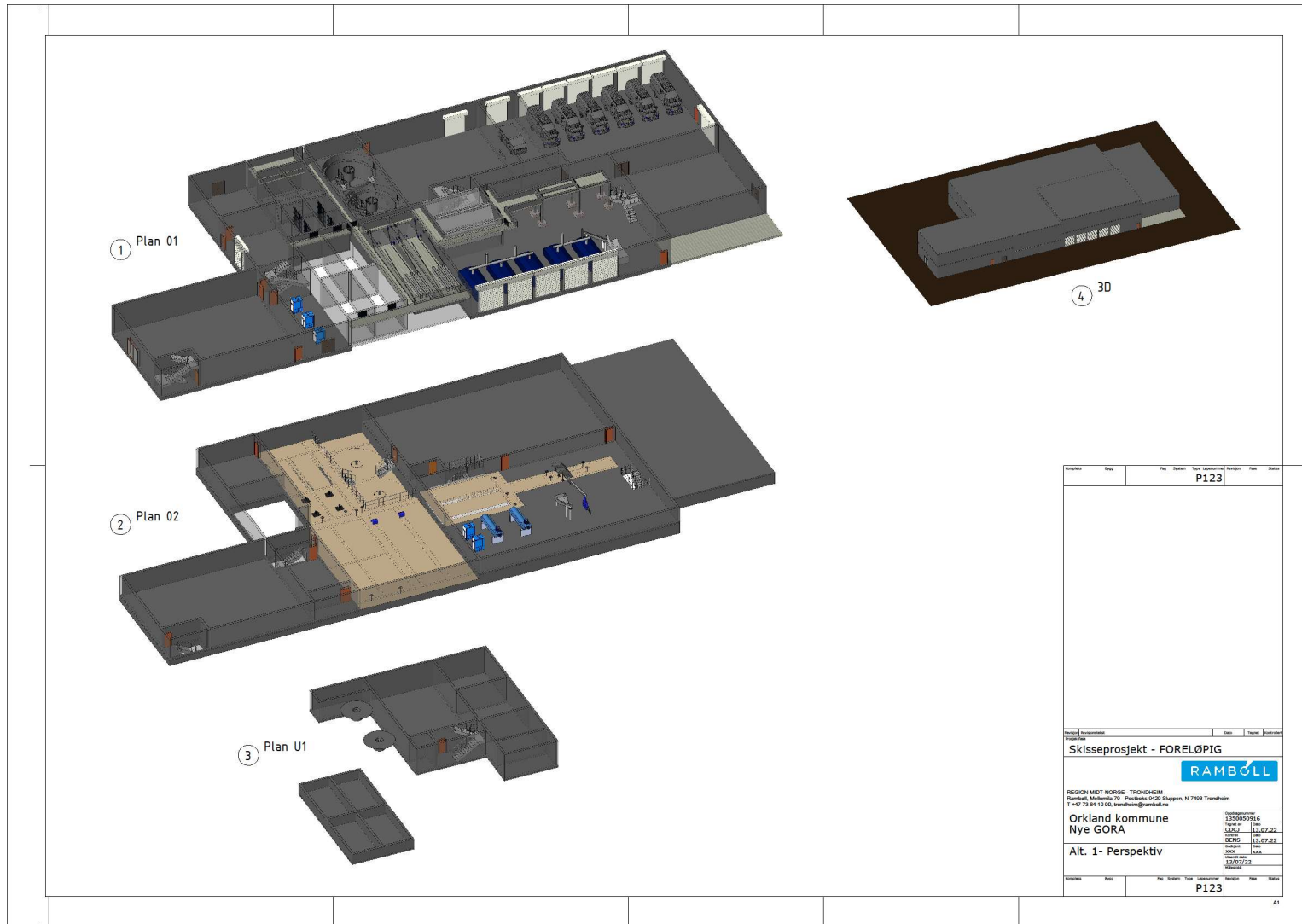
Figur 14 Planskisse for alternativ 1 med forsedimentering
