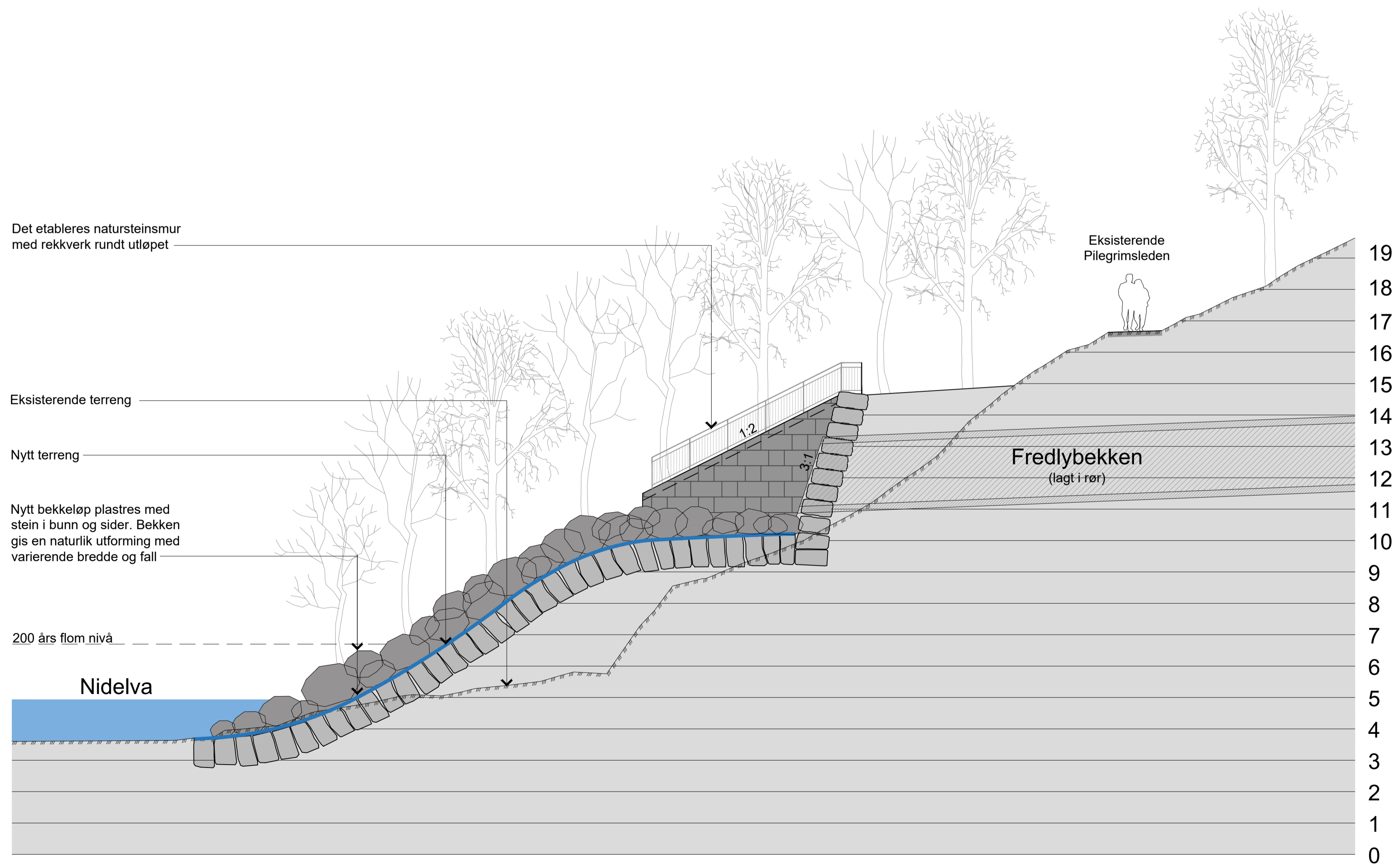
Snitt/oppriss B - B'
