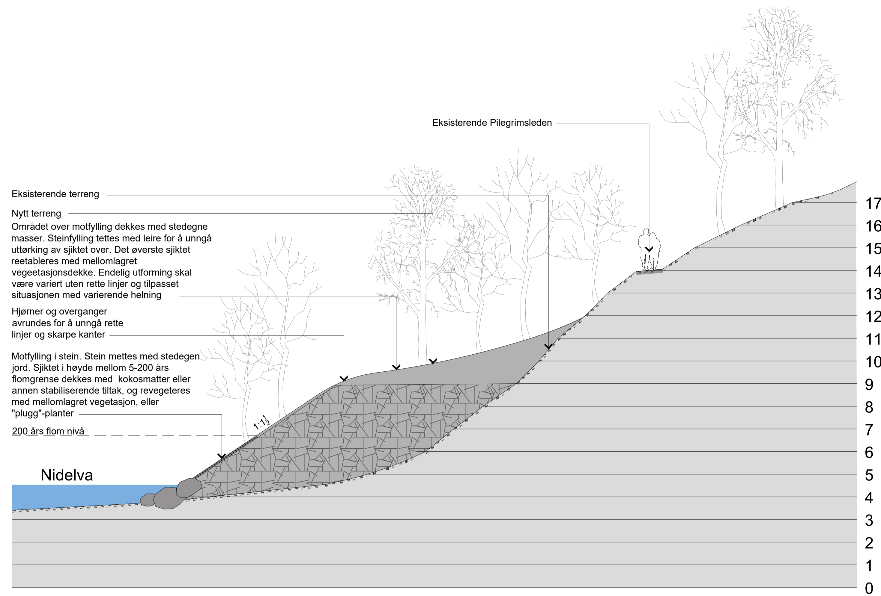
Terrengsnitt A - A'
