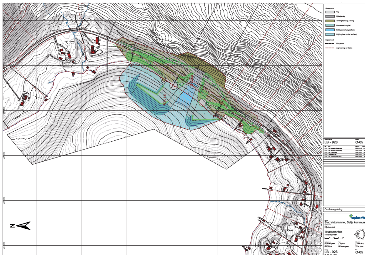
Figur 3-4. Stad tunnelen, entringsområde Moldefjorden. Tegning: Asplan Viak.
