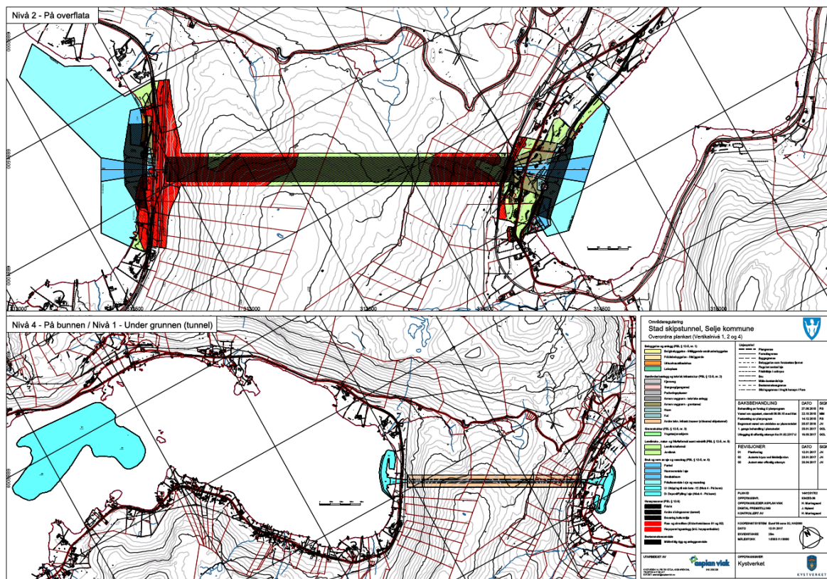
Figur 3-2. Stad tunnelen, plankart som viser entringsrådene i hhv. Moldefjorden og Kjødepollen, samt deponiområde for overskuddsmasser i Moldefjorden. Tegning: Asplan Viak.
