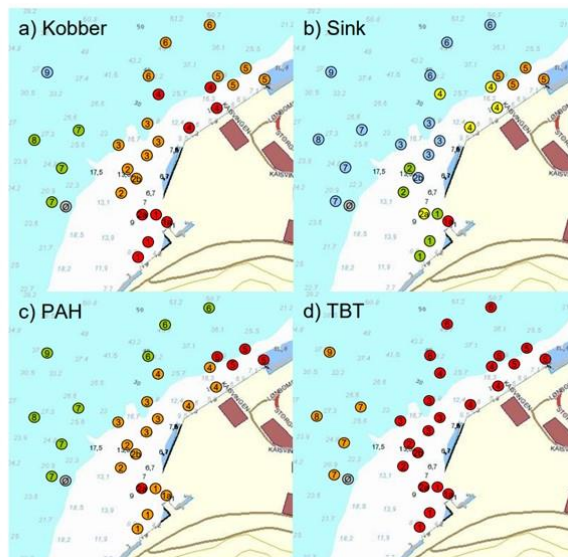
Figur 7. Til venstre: Resultater fra undersøkelser foretatt i 2008 utenfor Kimek AS. Til høyre: Kart som viser resultater av Kobber, sink, PAH og TBT ved prøvestasjonene farget etter tilstandsklasser (for beskrivelse av tilstandsklasser se Tabell 1).
