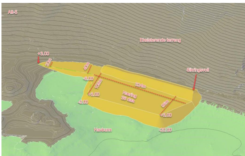
Figur 1 Skissert utfylling med dimensjoner, inkludert sikringsvoll og fyllingsfot. Kilde: Multiconsult
