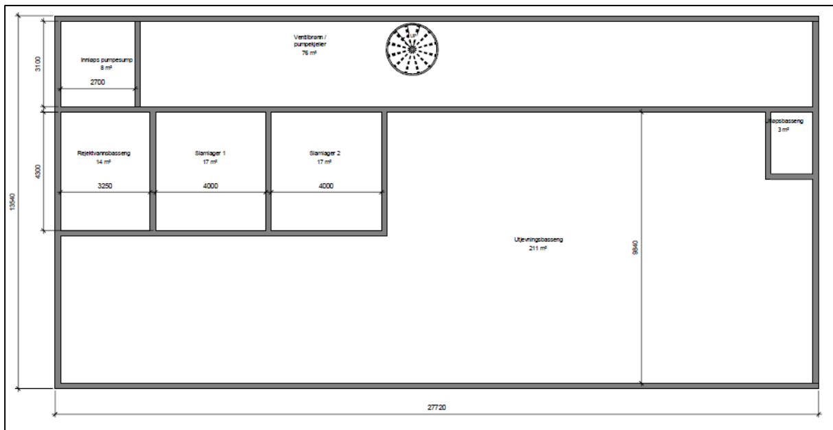
Figur 44. Foreløpig planskisse underetasje for RA i Nesbyen (Nesbyen + Nesfjellet) for 11 000 – 17 000 pe.
