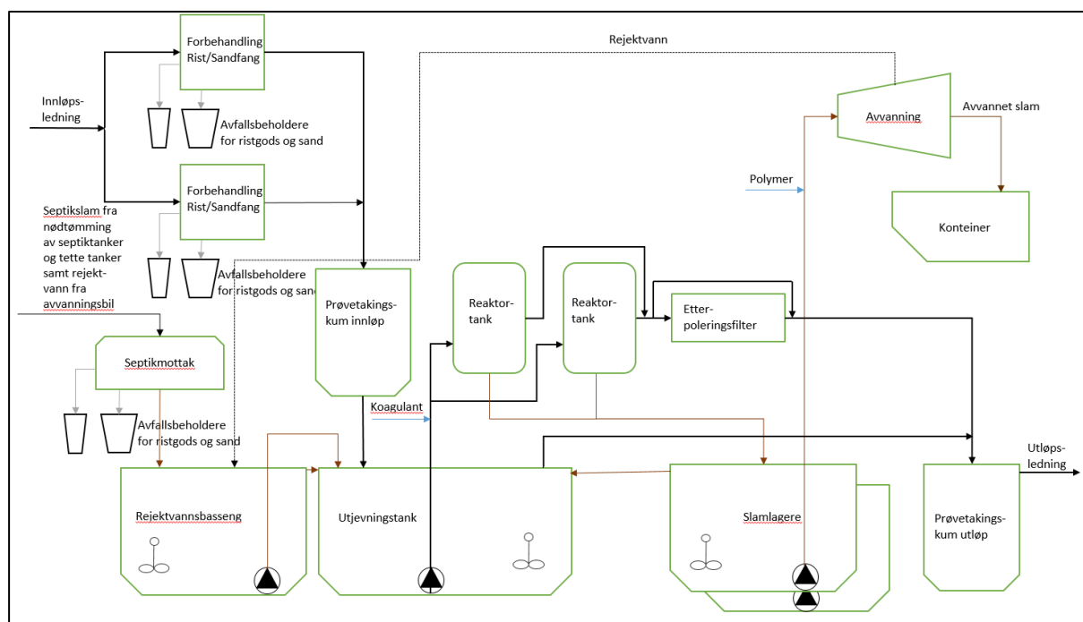
Figur 40. Flytskjema basert på SBR teknologi. Mulig renseprosessen på det nye rensanlegget i Nes kommune.
