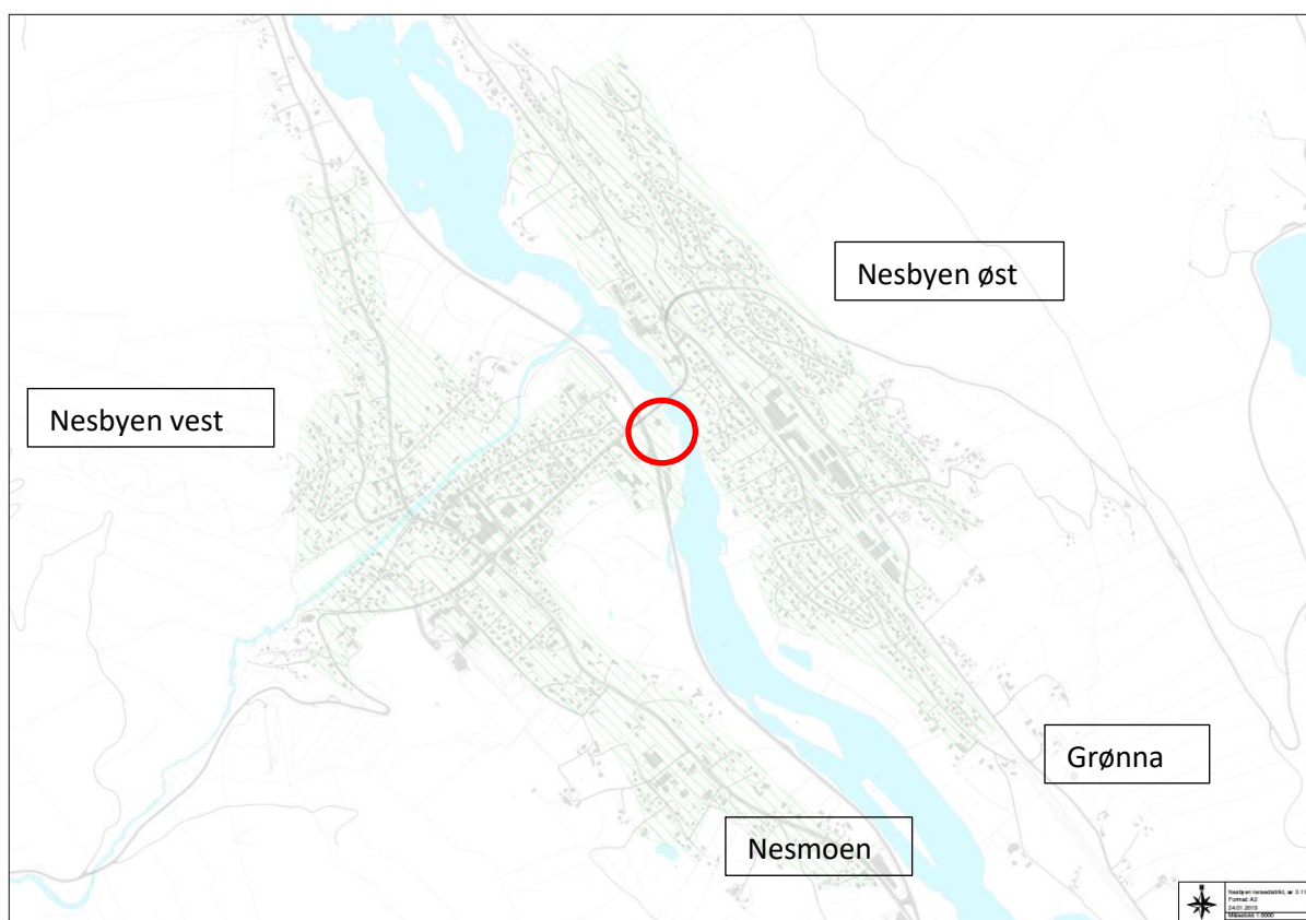
Figur 19. Kart over Nesbyen rensedistrikt fra 1990. Renseanlegg markert med rød sirkel. Områdene i sør er planlagt tilknyttet rensanlegget i relativt nær fremtid (Nesmoen og Grønna).
