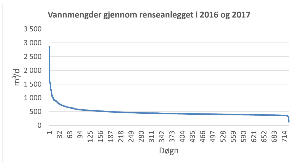
Figur 21. Varighetskurve for vannmengder til renseanlegget i 2016 og 2017.
