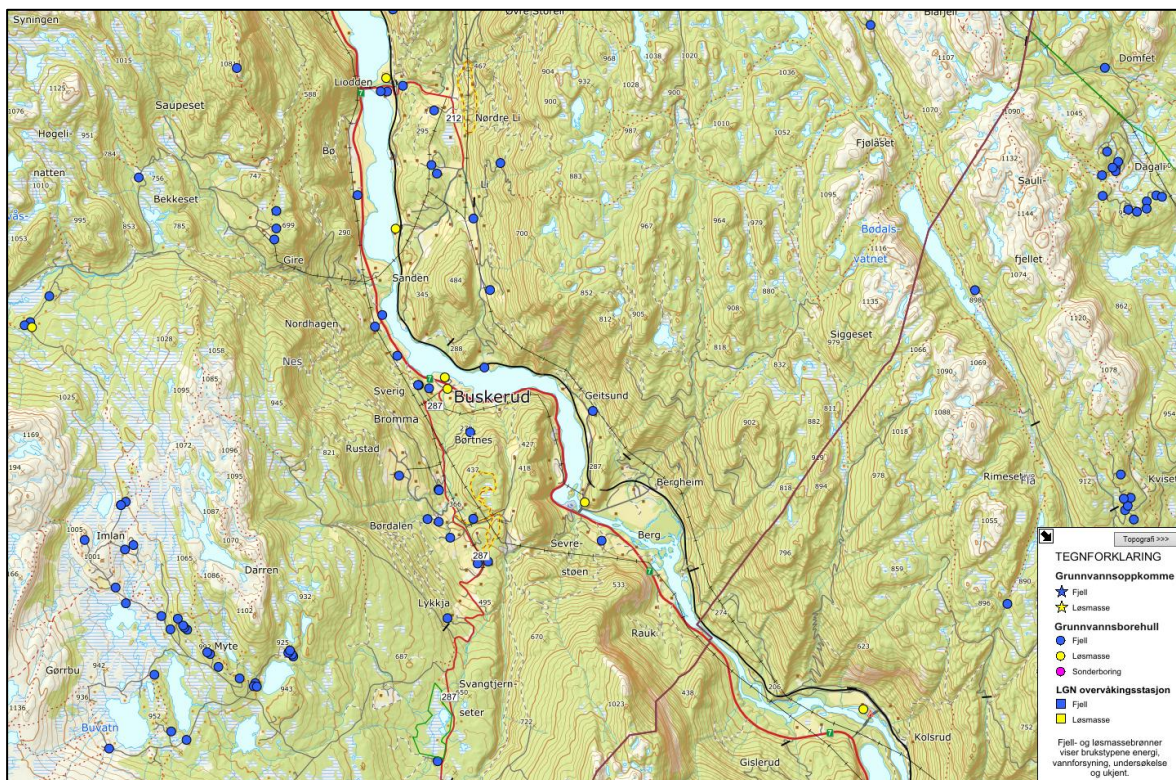
Figur 14. Registrerte brønner i fjell og løsmasser mellom Nesbyen og Flå. Borebrønner i løsmasser er markert med gul farge. Kilde: NGU brønn databasen Granada.
