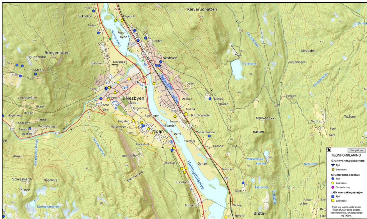
Figur 13. Registrerte brønner i fjell og løsmasser i Nesbyen. Det er flere borebrønner i løsmasser langsmed elva nedover langs Hallingdalselva. Kilde: NGU brønn databasen Granada.
