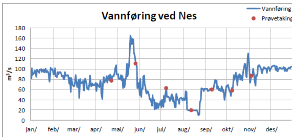
Figur 29. Vannføring ved Nes 2014. Røde sirkler markerer tidspunkt for uttak av prøver ved Melen som er nærmeste stasjon for prøvetaking. Tabellen er hentet fra Overvåking av Hallingdalsvassdraget i 2014.
