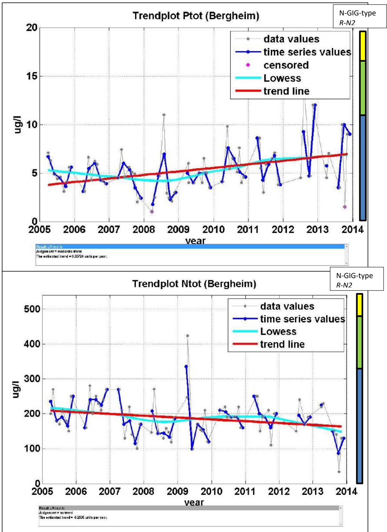
Figur 35. Trendplot med målinger av totalfosfor og totalnitrogen ved målestasjonen Bergheim. Hentet fra Årsrapport Hallingdalsvassdraget i 2013 (Rambøll, 2013).
