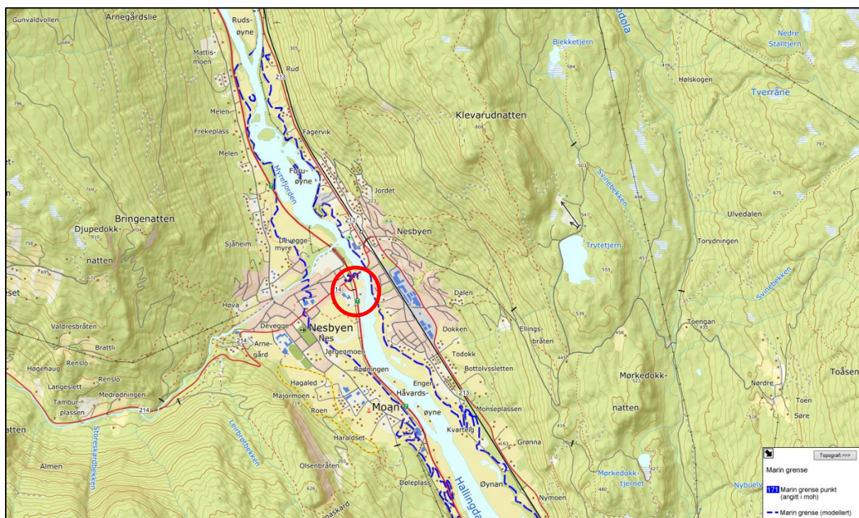
Figur 12. Nesbyen renseanlegg ligger under Marin Grense, som er markert med stiplet blå linje. Kilde: NGU.
