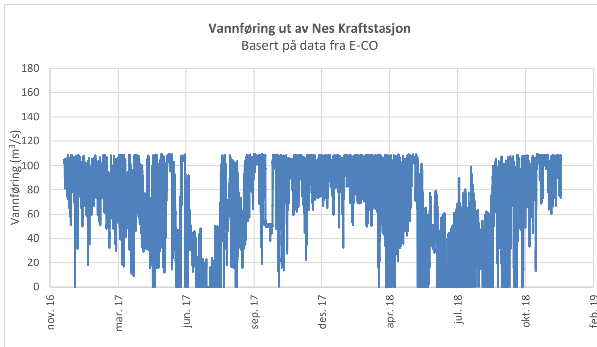
Figur 28. Vannføringsmålinger ut fra Nes Kraftstasjon fra desember 2016 til februar 2019.
