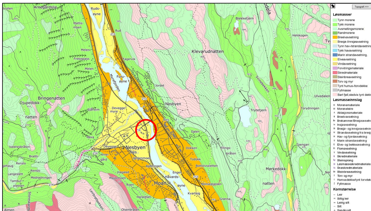
Figur 11. Nesbyen renseanlegg er lokalisert på en større vifteformet sand- og grusavsetning, avsatt av elva Rukkedøla ut i Hallingdal. Kilde: NGU løsmassekart.
