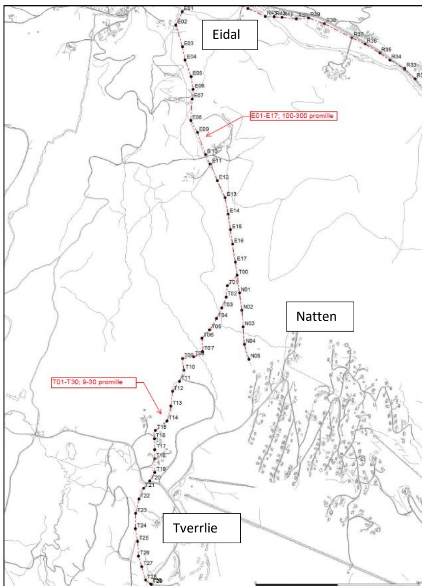
Figur 22. Oversiktstegning hovedledningsanlegg for Natten / Tverrlia området, fra Cowi rapport (2012).
