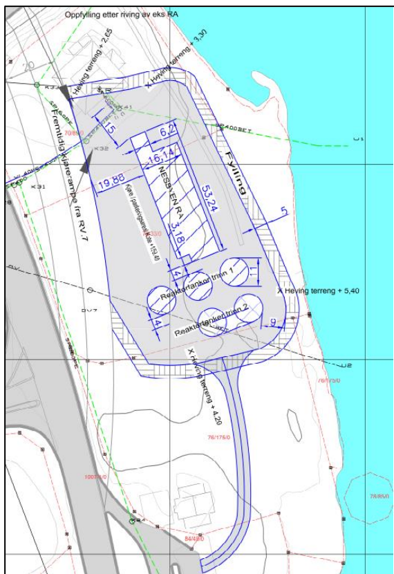
Figur 41. Foreløpig situasjonsplan for anlegg for 11-17 000 pe (Nesbyen + Nesfjellet) i Nesbyen.
