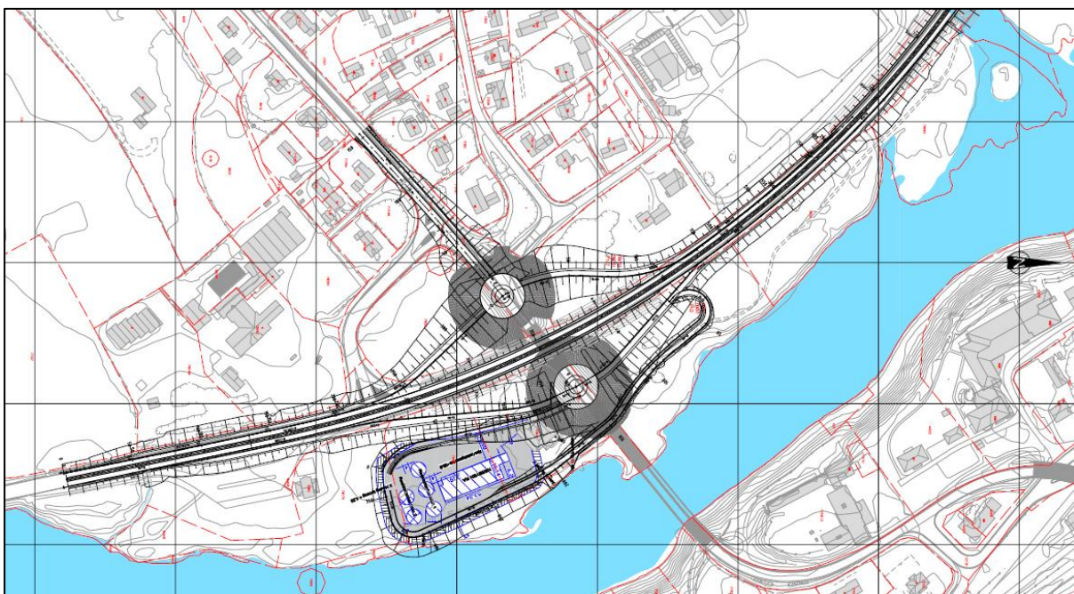
Figur 7. Foreløpig illustrasjon av mulig nytt renseanlegg og nye av- og påkjøringsramper til Rv 7.
