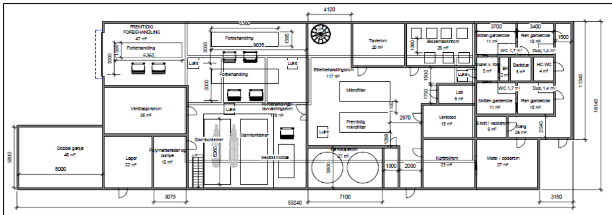
Figur 43. Foreløpig planskisse 1. etasje for RA i Nesbyen (Nesbyen + Nesfjellet) for 11 000 – 17 000 pe.
