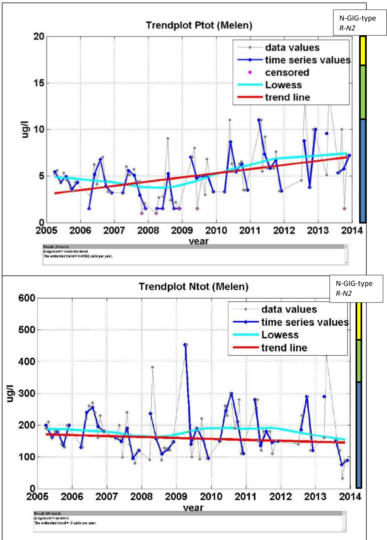
Figur 34. Trendplot for perioden 2005-2013 for fosfor og nitrogen ved målestasjonen Melen. Hentet fra Årsrapport Hallingdalsvassdraget i 2013 (Rambøll, 2013).
