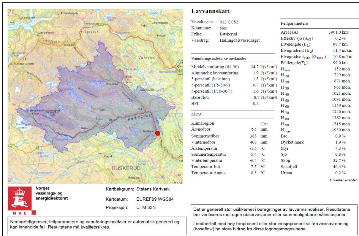
Figur 26. Lavvannskart generert av NEVINA (NVE) for nedbørfeltet oppstrøms Nesbyen renseanlegg.
