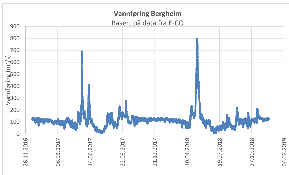
Figur 32. Vannføringsmålinger fra Hallingdalselva ved Bergheim. Målingene er basert på data fra E-CO.
