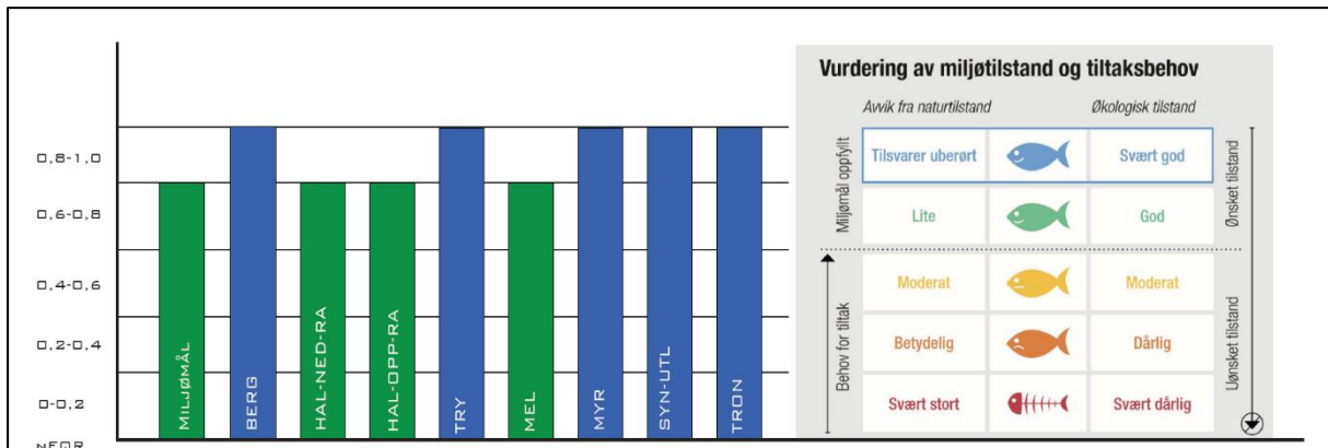
Figur 38. Normaliserte EQR-verdier for hver prøvestasjon og tiltaksbehov. Figuren er hentet fra Vassdragsovervåking i Hallingdal 2015-2017 (Faun naturforvaltning, 2018).
