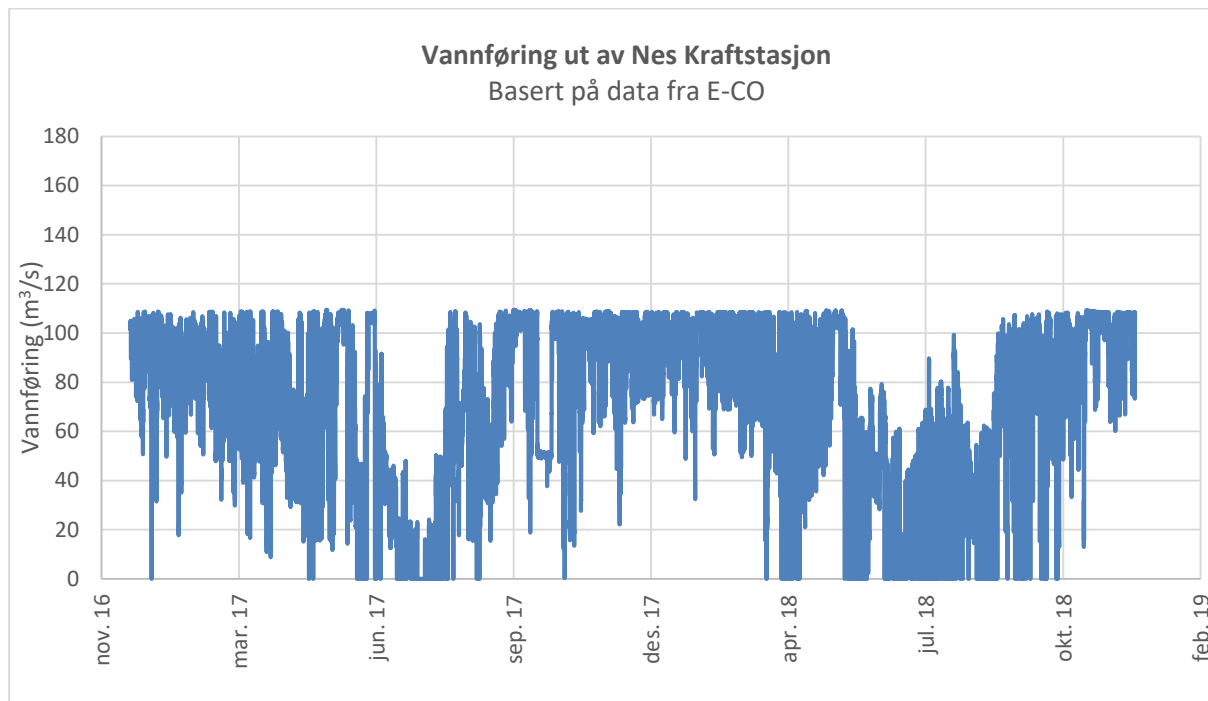
Figur 30. Vannføringsmålinger ut av Nes Kraftstasjon fra E-CO i perioden 2016 til 2018. Lavest vannføring er målt i juli 2017 og 2018.
