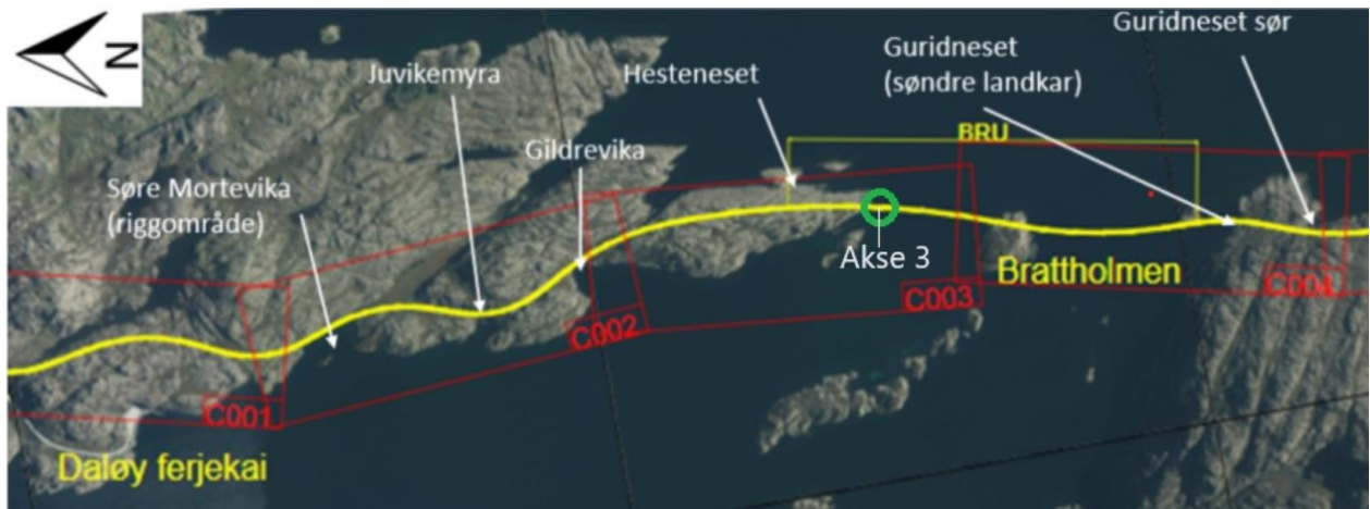
Figur 1 Brufundamentet som skal beskyttes (akse 3) er markert med grønn sirkel
