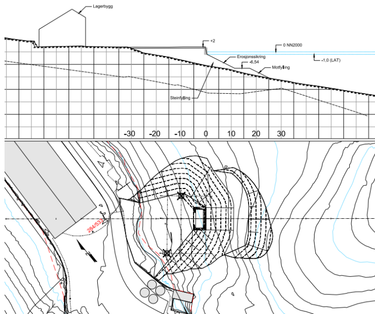
Figur 1 Garnes kaihakk, plan og snitt Multiconsult
