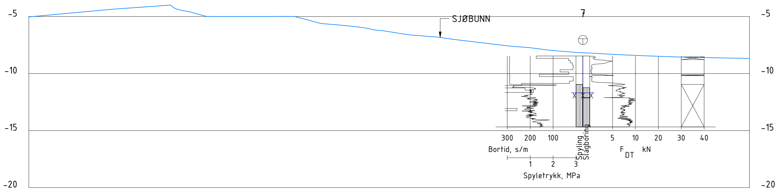
Profil B-B
