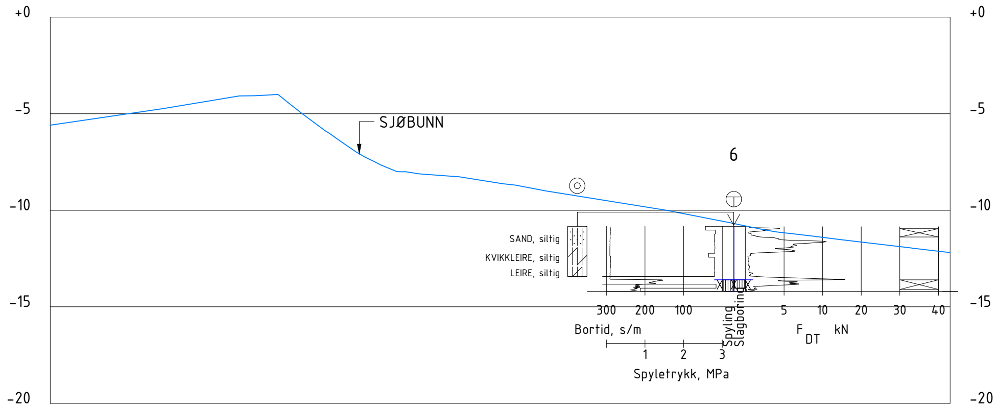
Profil C-C
