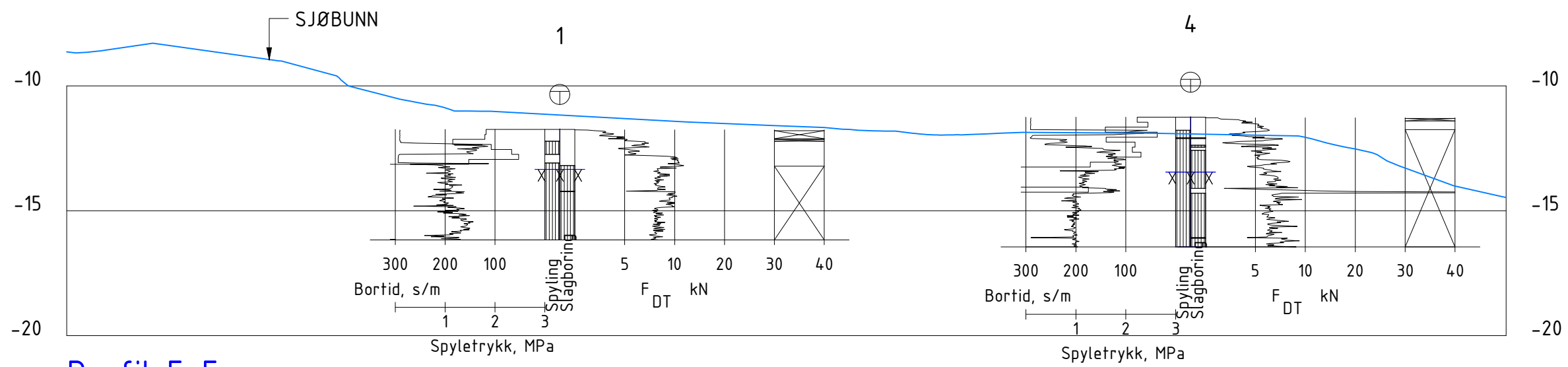
Profil E-E
