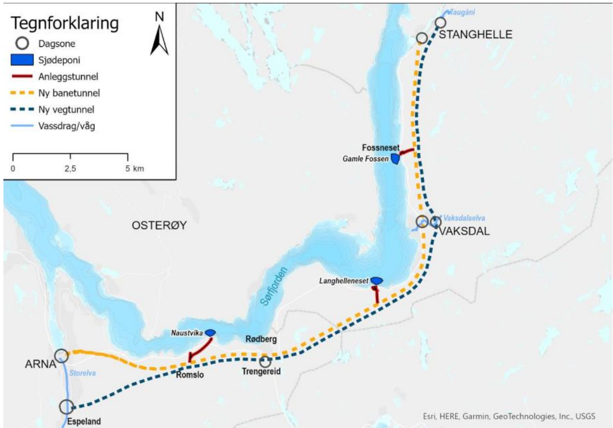
Figur 1 Det er planlagt anleggstunnelar og riggområder ved Fossneset og Gamle Fossen, Langhelleneset, Romslo og Naustvika nær Sørffjorden i FAS. I tillegg er det planlagt utsleppsleidningar for tunnelvann ved Gamle Fossen, Langhelleneset, Trengereid og Romslo. Utsleppet frå Trengereid inngår i søknad Midt
