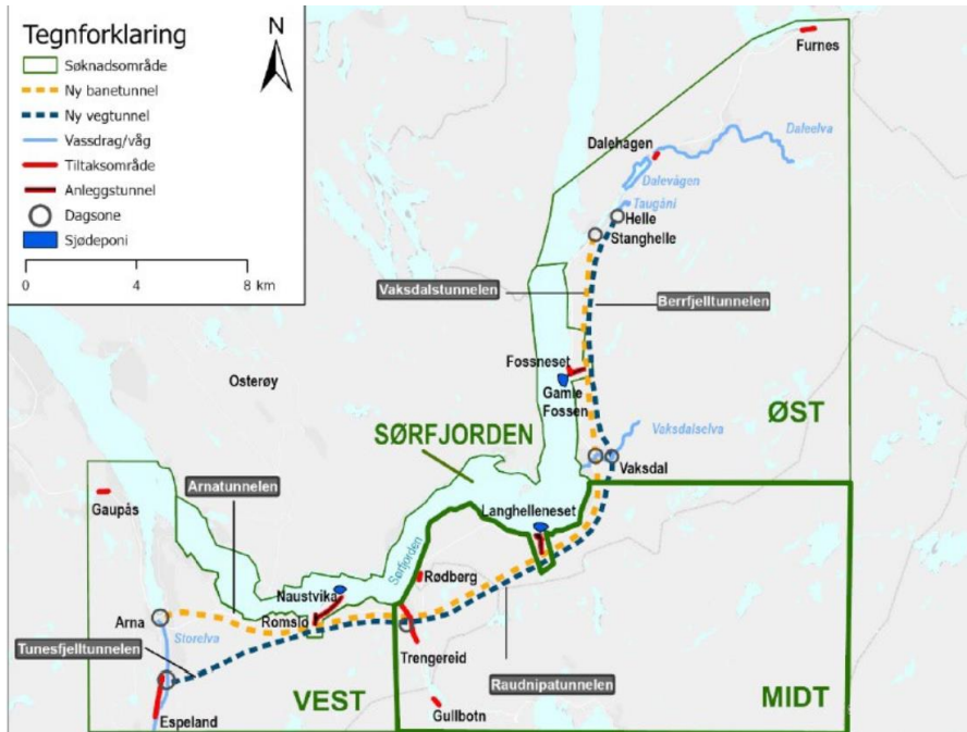
Figur 2 Oversikt inndeling i søknadsområde Vest, Midt, Øst og Sørkjolen, Kjelde: Statens vegvesen
