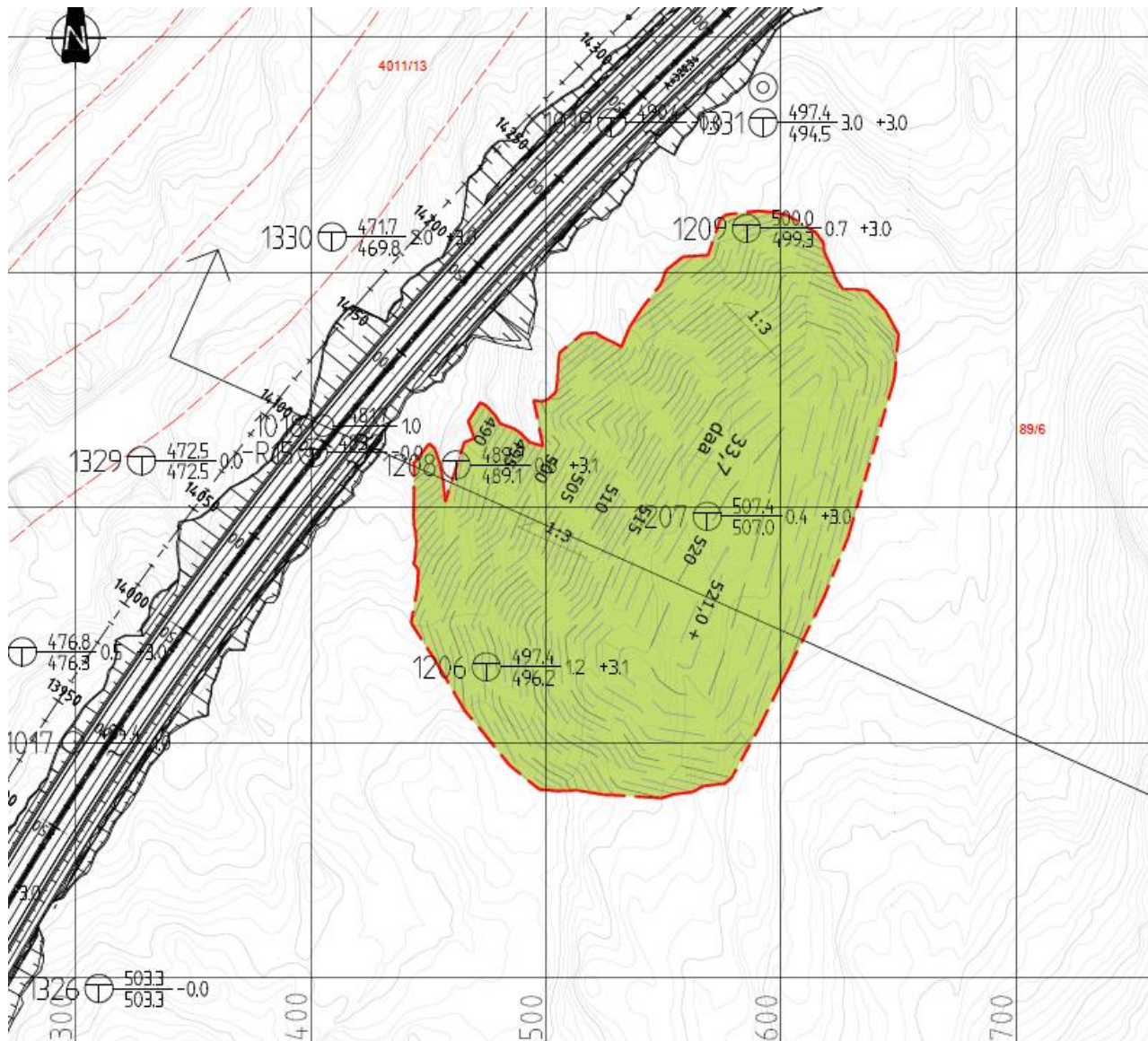
Figur 9: Utsnitt fra situasjonsplan med borpunkter ved BAA4 (kilde: Rambøll).
