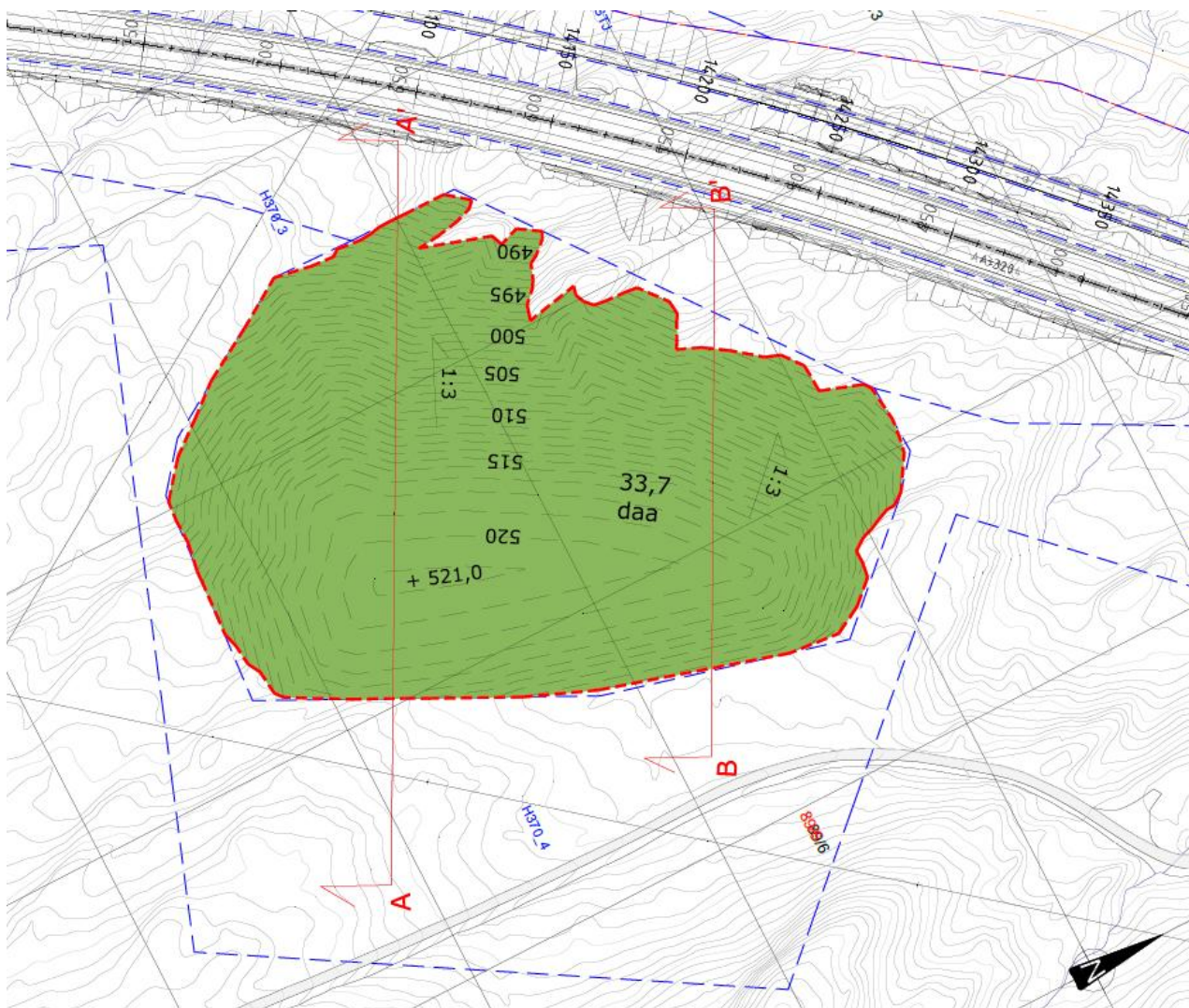
Figur 10: Utsnitt fra landskapsplan massedeponi BAA4, tegning O-011, foreløpig, 7.1.2021 (kilde: Rambøll).
