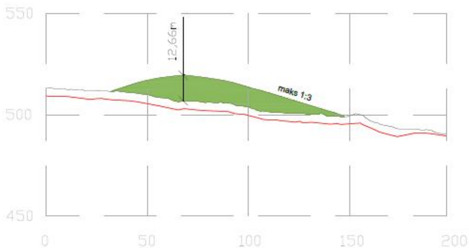
Figur 11: Utsnitt fra landskapsplan massedeponi BAA4, tegning O-011, foreløpig, 7.1.2021 (kilde: Rambøll).
