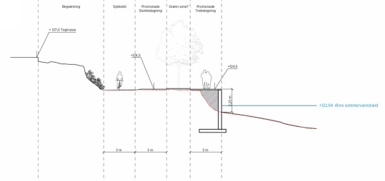
Snitt AA
