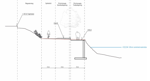
Snitt BB
