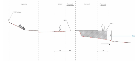
Snitt DD
