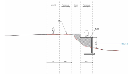
Snitt EE
