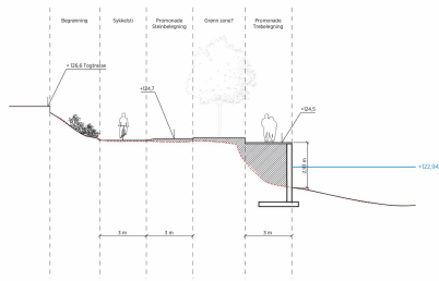
Snitt CC
