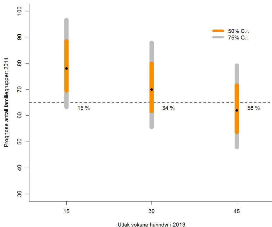
Figur 9. Prognose for antall familiegrupper på landsbasis før jakta i 2014 gitt tre ulike senarioer for uttak av voksne hunddyr under jakta i 2013 (henholdsvis 15, 30 og 45 voksne hunddyr). Sannsynligheten for å falle under bestandsmålet på 65 er hhv 15 %, 34 % og 58 % for de tre senarioene. Punktestimertene (sort prikk) er hhv 79, 70 og 62 familiegrupper. Orange strek angir 50 % C.I. og sort strek angir 75 % C.I. Stiplet horisontal linje angir bestandsmålet på 65 familiegrupper (NINA Rapport 859)
