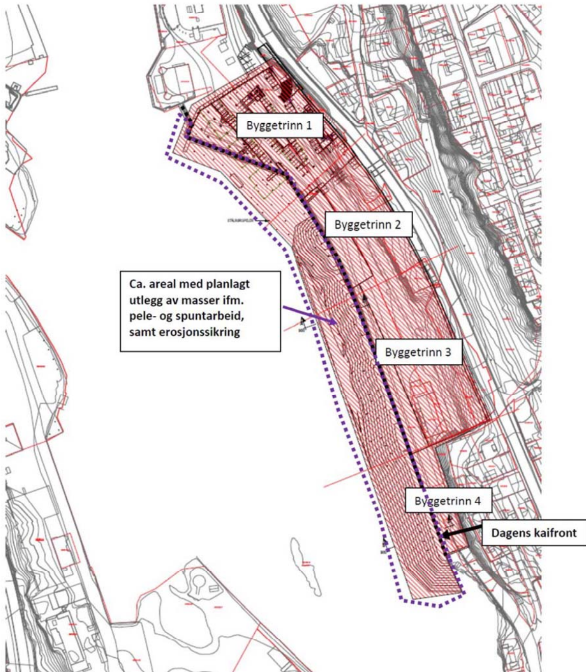
Figur 1: Planlagt areal i elva som berøres av masseutlegg samt pæle- og spuntarbeidene (grunnlag: Kruse Smith Entreprenør AS)
