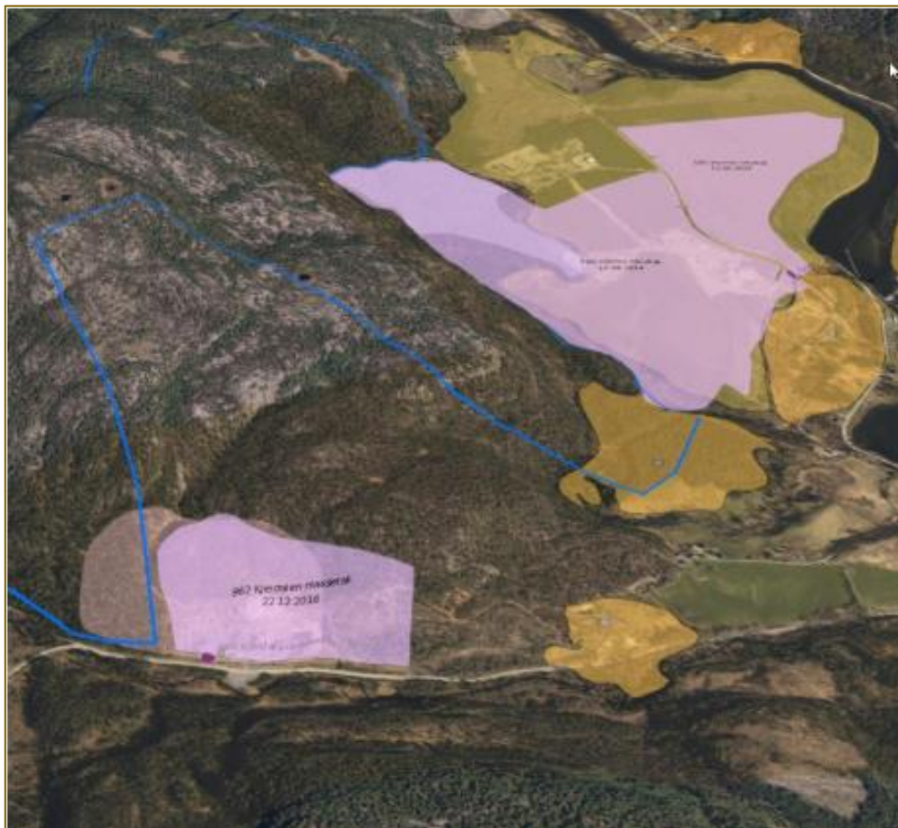
Figuren viser konsesjonsområde etter minerallova § 43 (rosa), sand- og grusforekomstar (oransje) og pukkforekomstar (gjennomsiktig lys rosa).
